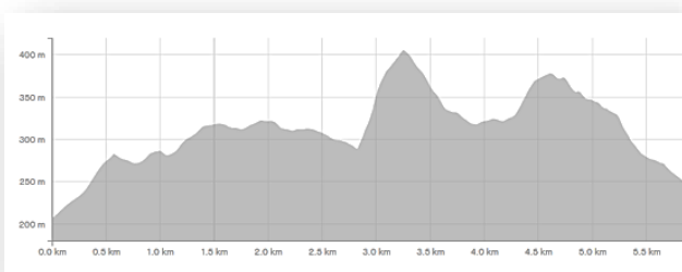
5.9k elevation
